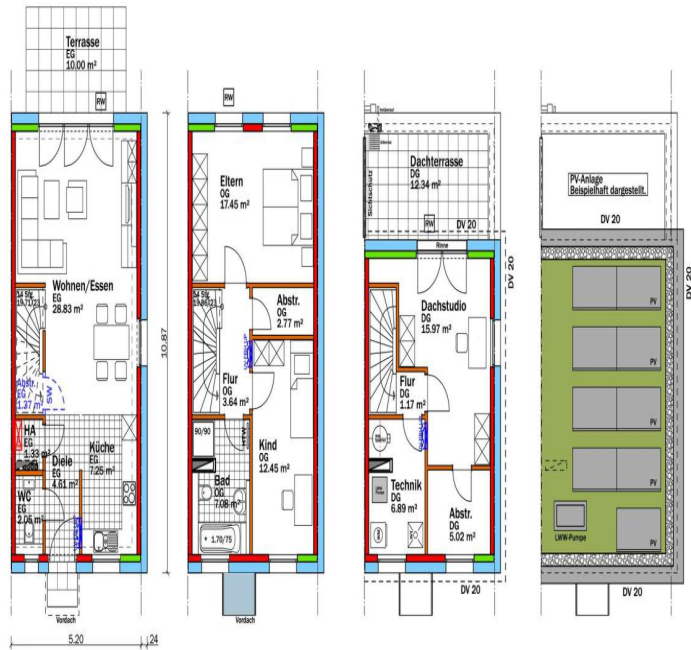
Erdgeschoss Obergeschoss Dachgeschoss Dachaufsicht
