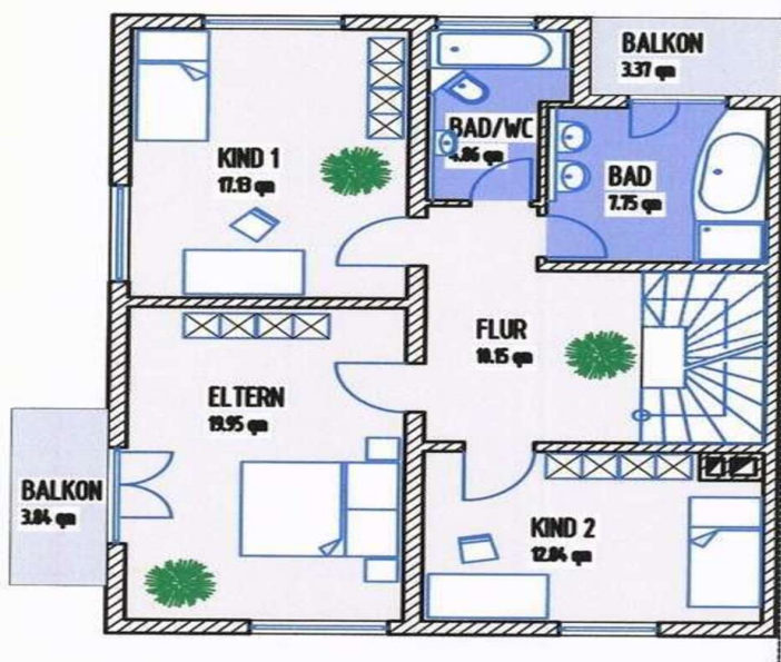
OBERGESCHOSS
