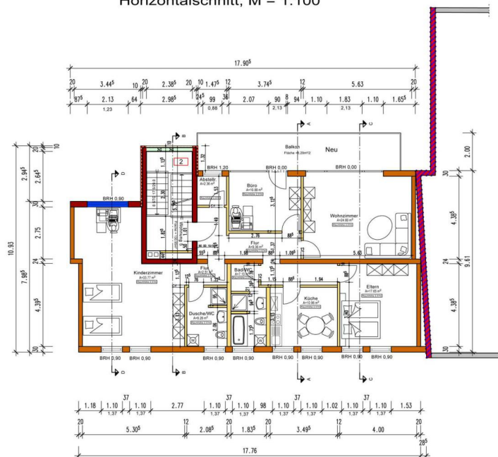
Horizontalschnitt, M = 1:100
