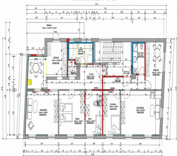
Grundriss Obergeschoss Horizontalschnitt, M = 1: 50
