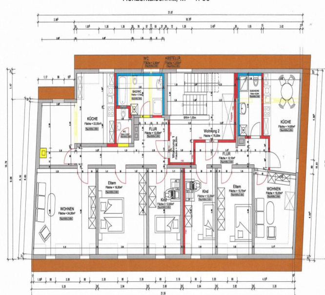
Grundriss Dachgeschoss Horizontalschnitt, M = 1: 50
