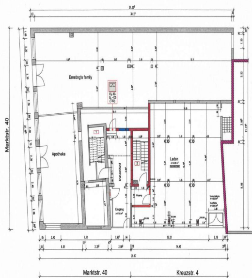
Grundriss Erdgeschoss
